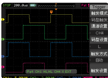
码型触发
